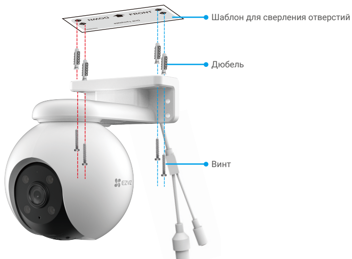
Рисунок 1. Монтаж на потолок
